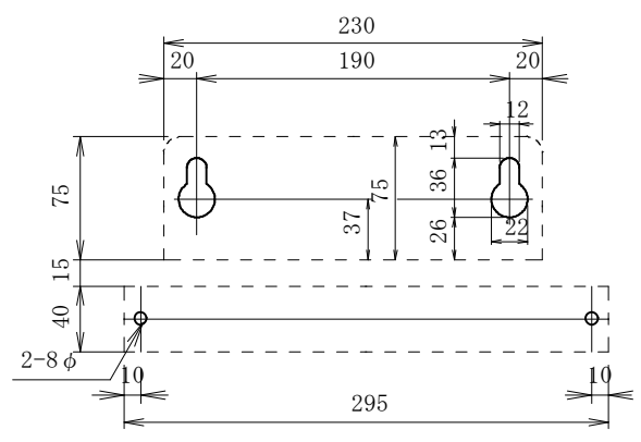
取付プレート穴位置 (S : 1 / 5)
